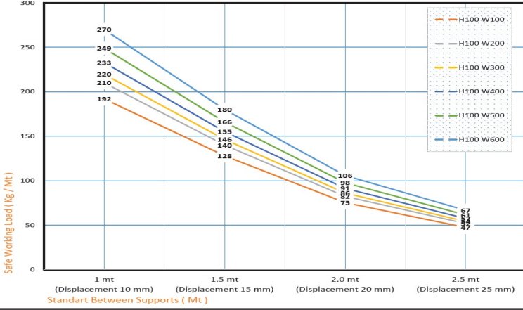
H100 ALL SERIES CABLE TRAY LOAD GRAPH (TS EN 61537)
